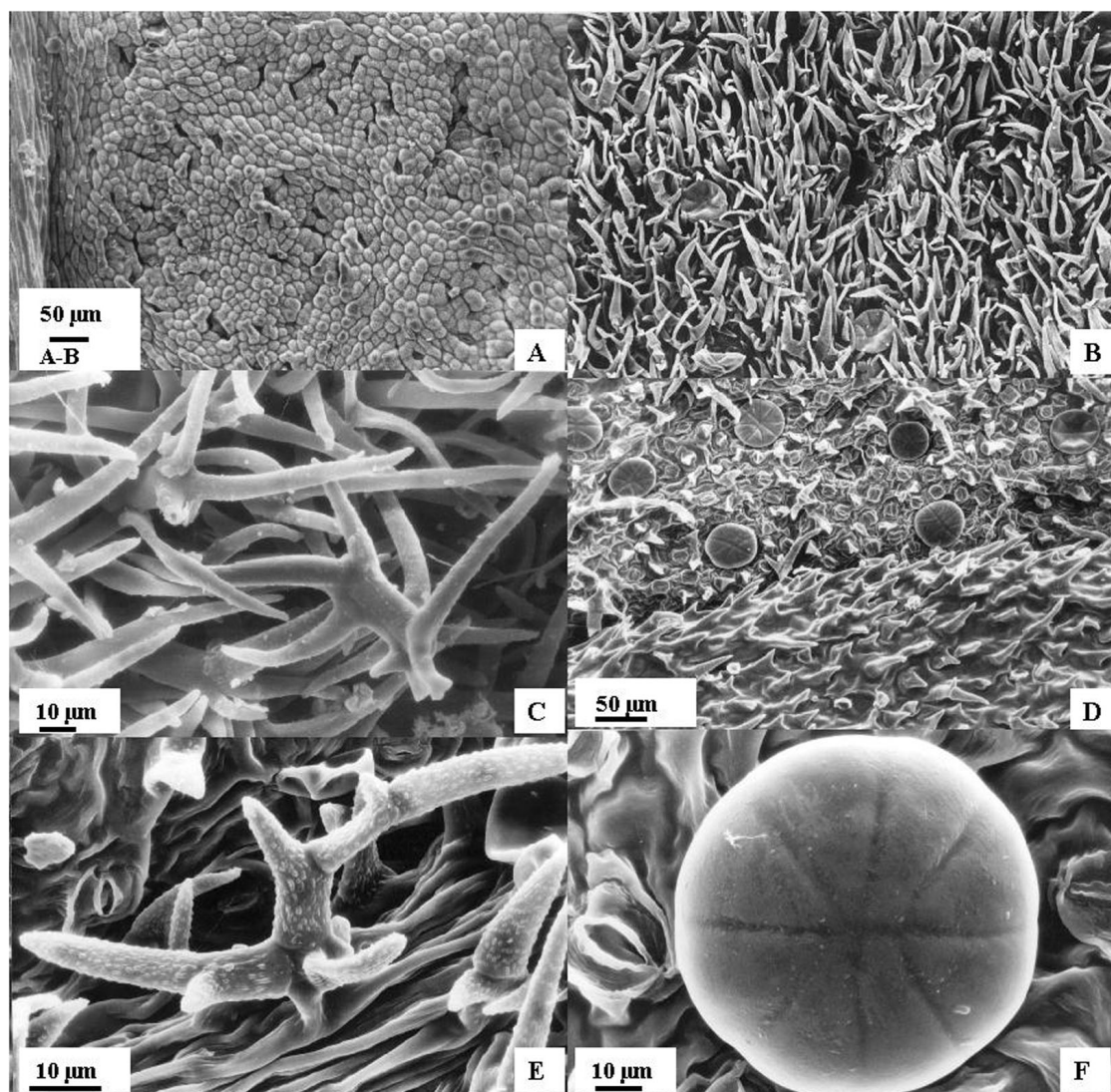
Fig. 2. Micromorfología foliar de Cunila . A , C. angustifolia vista general de la epidermis abaxial con estomas anomocíticos. B-C , C. incana . B , vista general del indumento con pubescencia densa, tricomas glandulares y no glandulares en cara adaxial. C , detalle de tricomas no glandulares pluricelulares ramificados de superficie lisa. D-F , C. microcephala . D , detalle de la nervadura media en cara abaxial con tricomas pluricelulares y glándulas secretoras. E , detalle de un pelo pluricelular ramificado con superficie verrucosa. F , detalle de una glándula secretora con cabezuela de ocho células. A , de Pabst 6231 & Pereira 6494; B , de Schinini 5475; C , de Pedersen 9221; D-F , de Troncoso et al. 2463.
